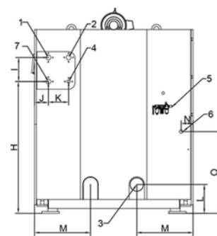
Вид сзади
