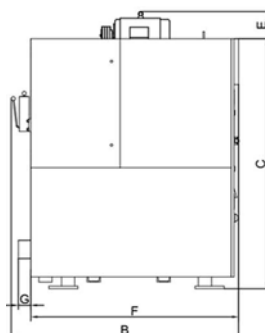
Вид сбоку
